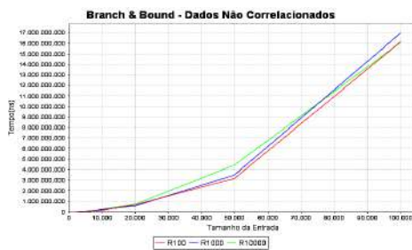
Figura 4: Comportamento do Branch and Bound
