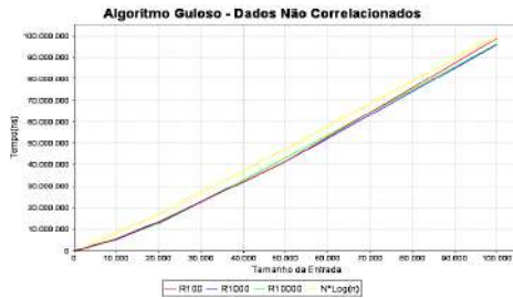
Figura 3: Comportamento do Algoritmo Guloso
